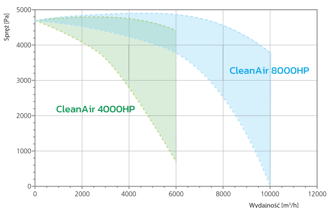
charakterystyka przepływu
