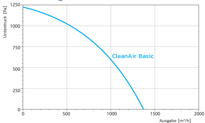
Leistungskurve
